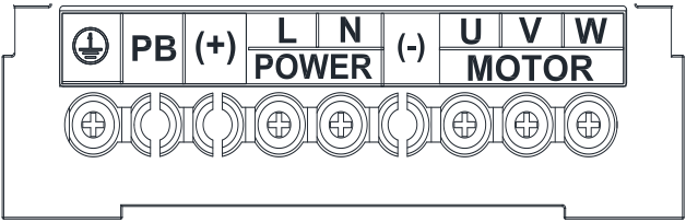
图 1-3 FR150A 单相主回路端子
