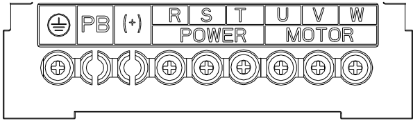
图 1-4 FR150A 三相主回路端子
