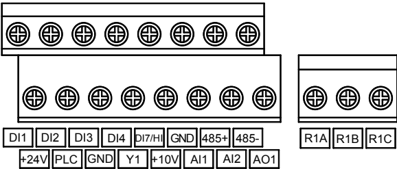
图1-5控制端子示意图
