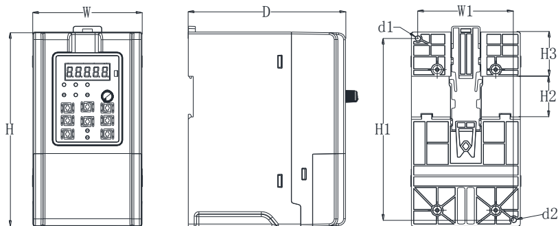
图 1-2 产品尺寸图
